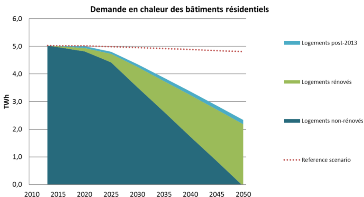
Figure 15. Evolution des besoins en chauffage dans les bâtiments résidentiels (Scénario -95%)
